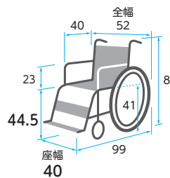
従来の標準車椅子フレーム
