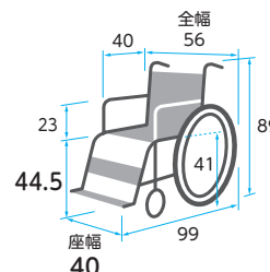
従来の標準車椅子フレーム
