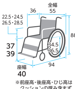
フットサポート 前後 & 角度調節
